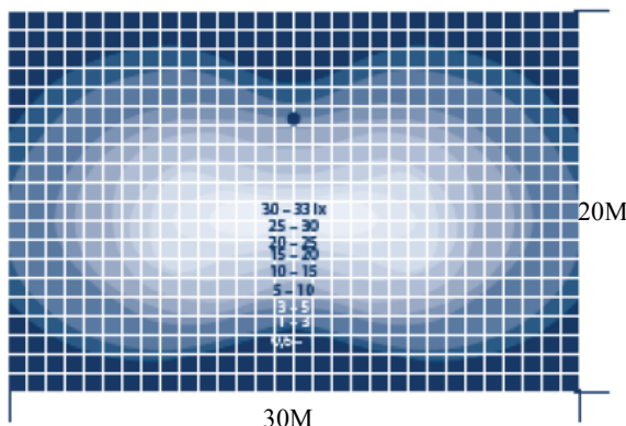
燈光分佈：橫向 裝燈高度：5.5 M
